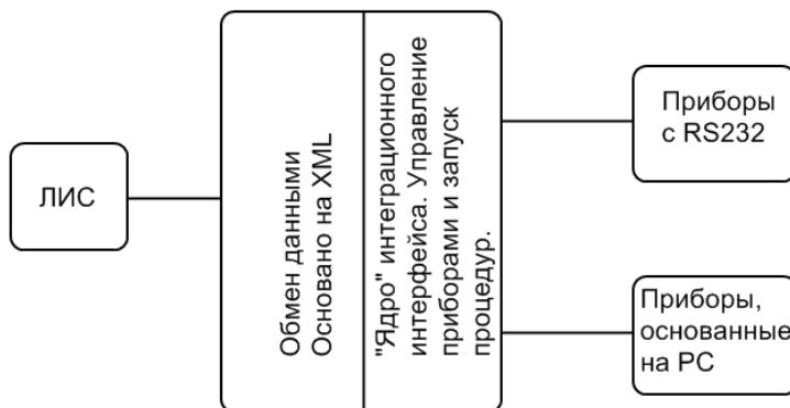
Рис. 1. Взаимодействие ЛИС и интеграционного интерфейса
